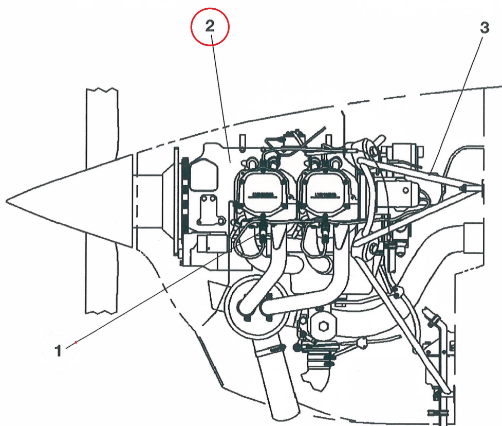
VIEW A-A
