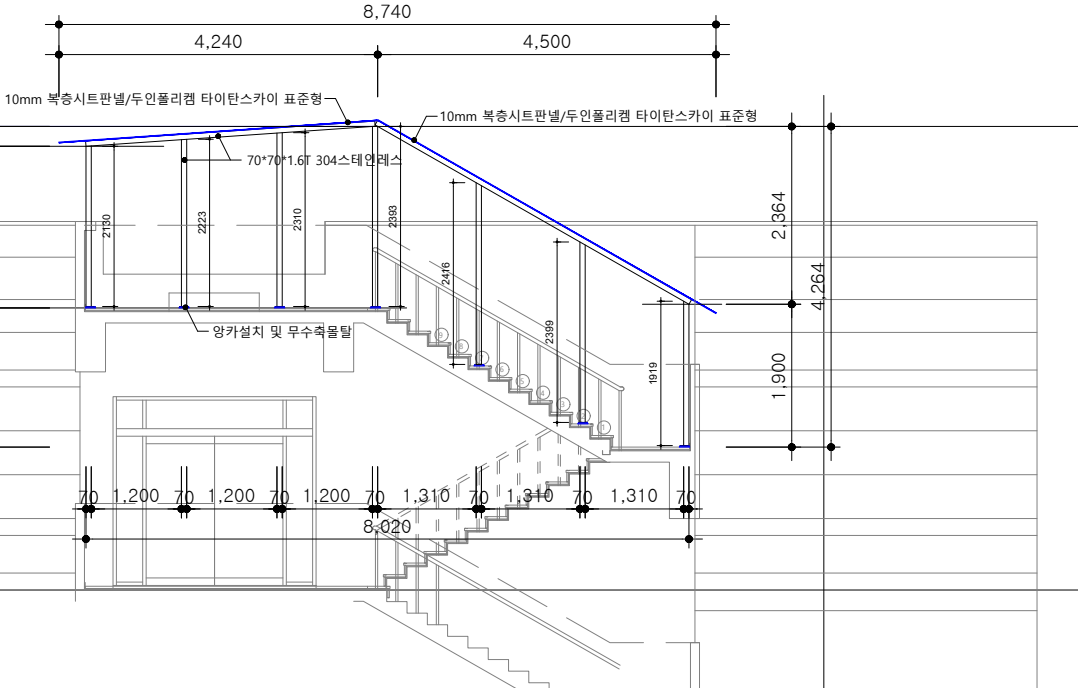
4 과학관 ROOF층 계단 단면도 축척 : 1/50
