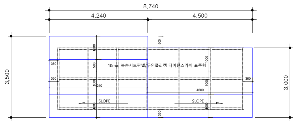
3 과학관 ROOF층 계단평면도 축척 : 1/50
