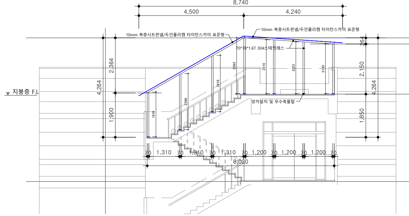
2 전자관 ROOF층 계단 단면도 축척 : 1/50
