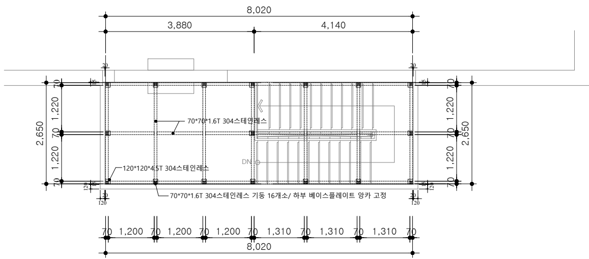
1 전자관 ROOF층 계단평면도 축척 : 1/50
